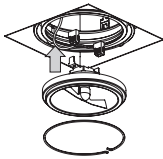
MITO 150 QR-LP111 with Accesories OPTION II
