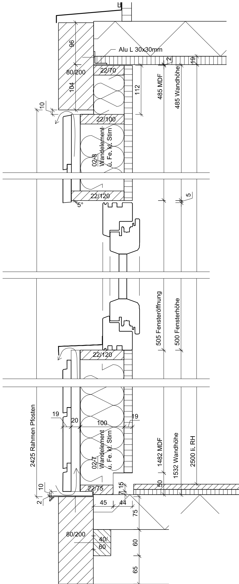
Fenster klein Stirn, Schnitt, 1:5
