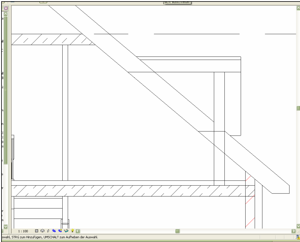
Schnitt A-A
