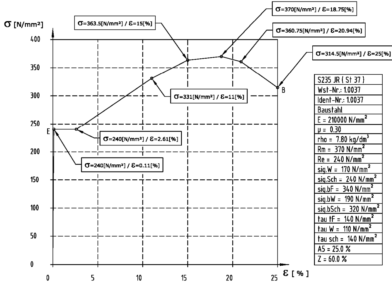
Spannungs-Dehnungs-Diagramm S235 JR
