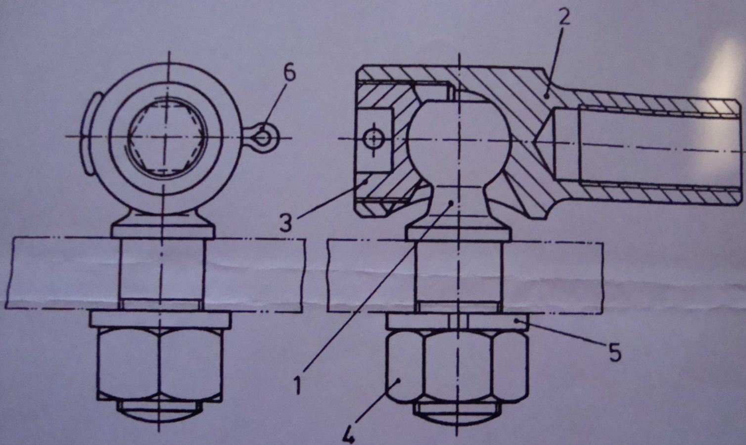
Abb. D.2: Kugelgelenk
