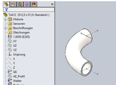
Rund-Stahlrohr gebogen (abgel. Konfi. vor Biegen)
